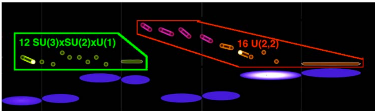
8 Fermion AntiParticles
