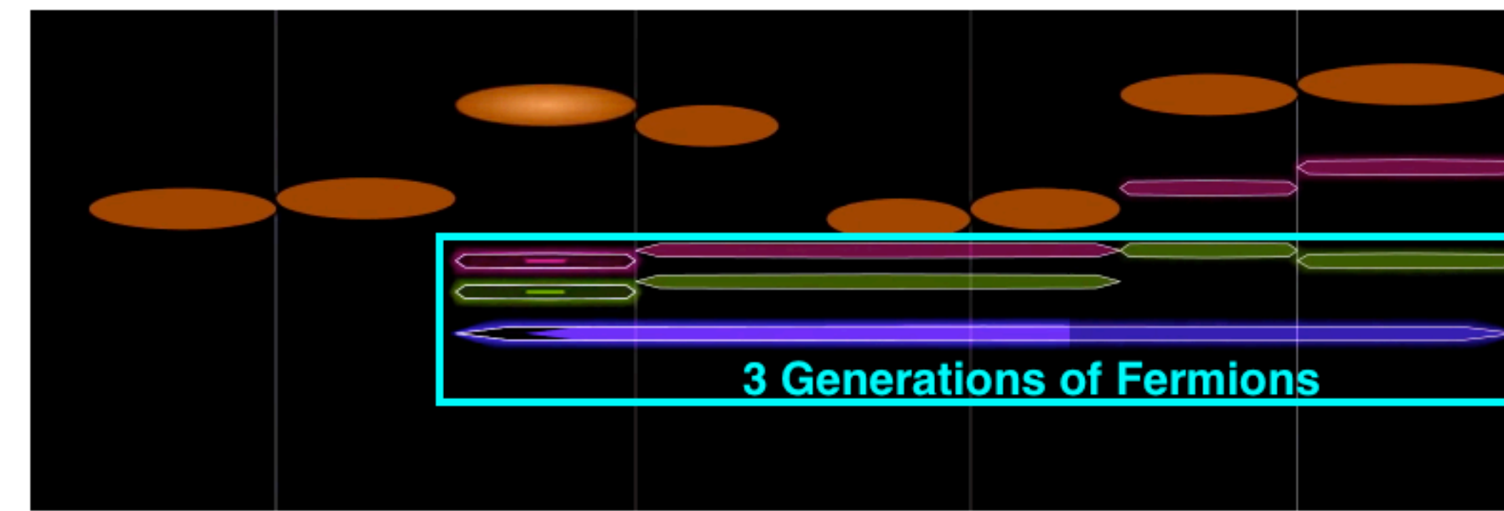
8 Fermion Particles
