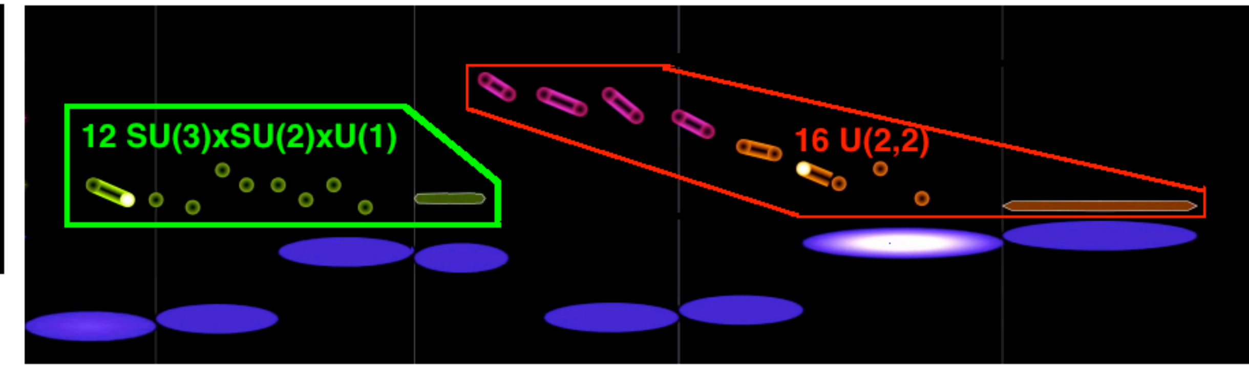
8 Fermion AntiParticles
