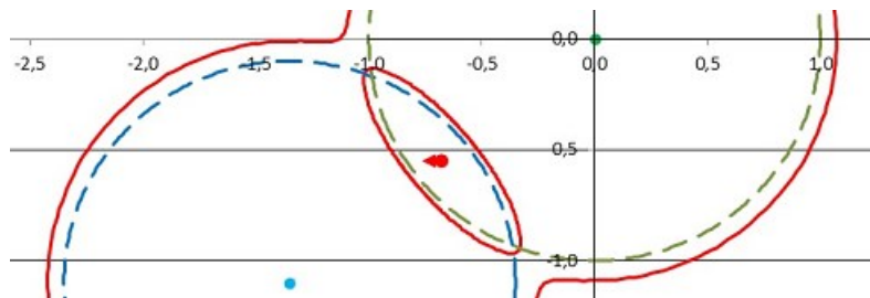
Рис.4 Через некоторое время движения двух сверхмассивных черных дыр полость внутреннего горизонта перемещается на другую сторону
