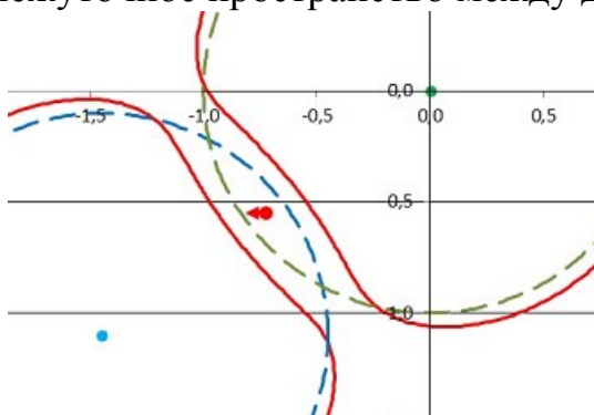
Рис.5 Две сверхмассивные черные дыры разошлись и образовали тоннель убежания
