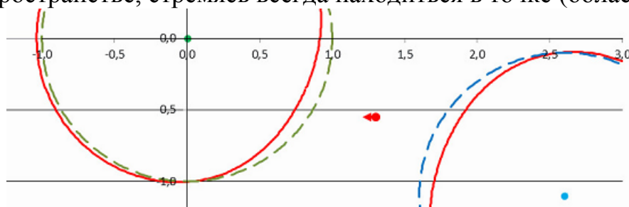
Рис.2 При сближении двух сверхмассивных черных дыр космолёт всегда должен находиться внутри области Лагранжа (вблизи тоннеля убегания)
